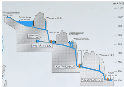
Längsschnitt Kraftwerke Schluchsee
